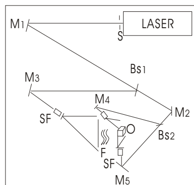
· 雙物光反射式全像術裝置
