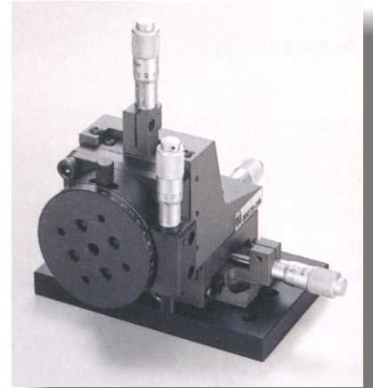
X, Y, Z, \theta_z , \alpha Axis 軸座
