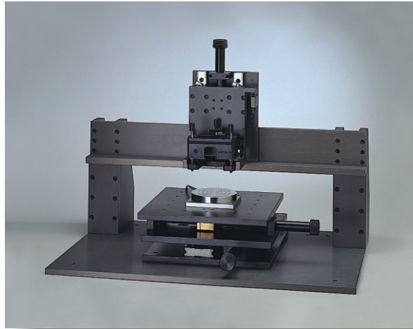
Wafer試驗系統
